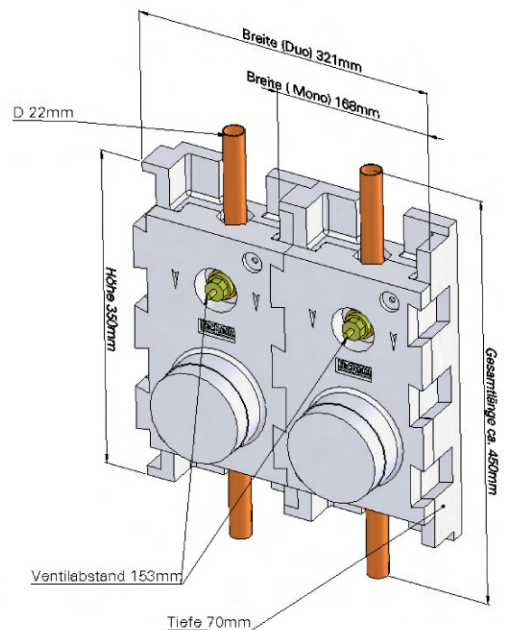
Montageblock mit Anschluss Löt/Press 22 mm
