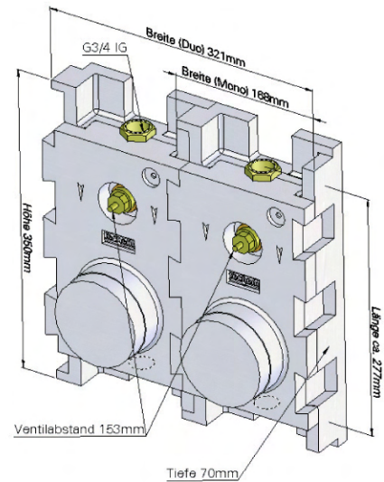
Montageblock mit Anschluss Innengewinde 3/4"
